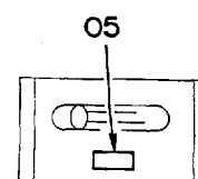
ロックレバーブラケット上面 UPSIDE VIEW OF LOCK LEVER BRACKET (4 本式レバー用) (FOR 4-LEVER TYPE)
