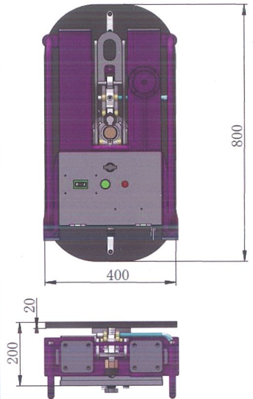
Glass boy-1-750k外观尺寸图
