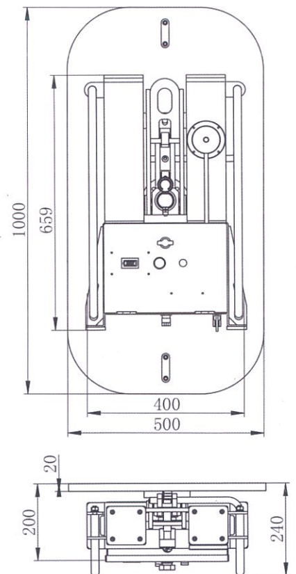
Glass boy-1-750k外观尺寸图
